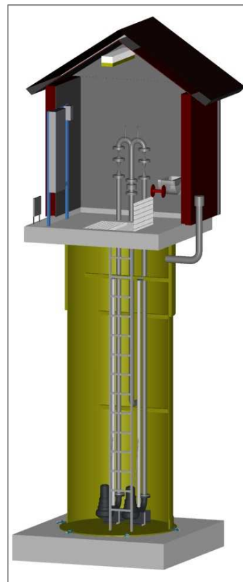
КНС с павильоном
